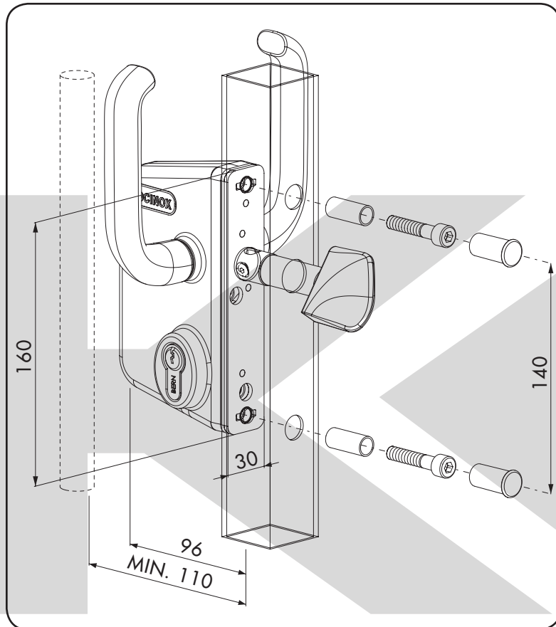
③ P ěprava profilu pro LSKZ U2
