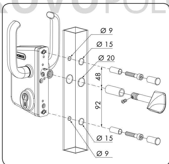
③ P ěprava profilu pro LSKZ U2
